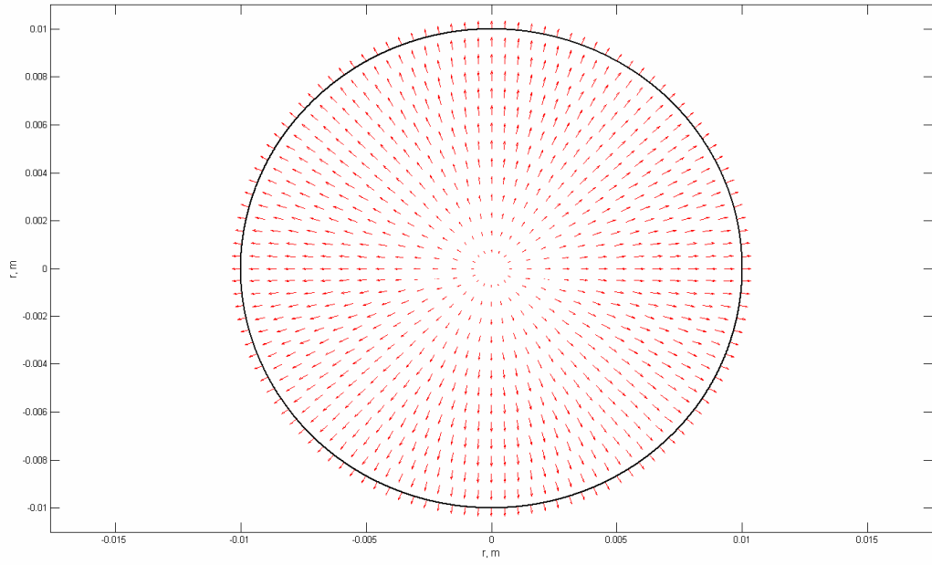
E_{01} , elektrinis laukas, z=\lambda/4
