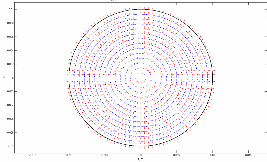
E_{01} , elektrinis ir magnetinis laukai, z=\lambda/4
