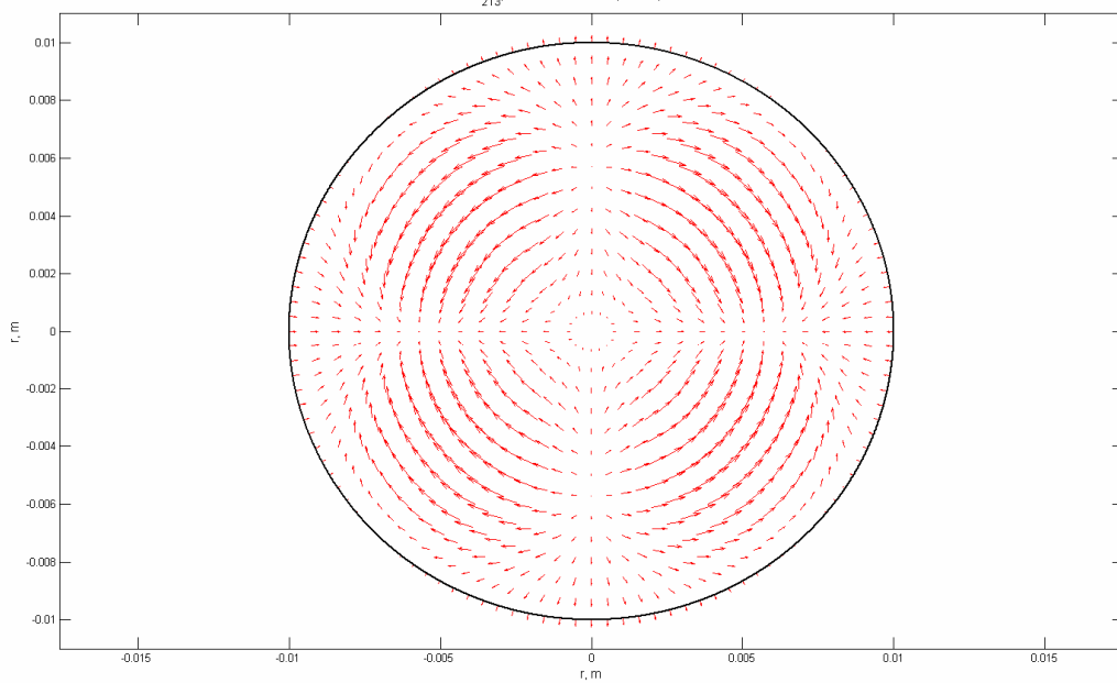
E_{z13} elektrinis laukas, z=l/2 , t=T/Inf
