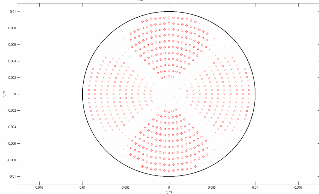
E_{z13} elektrinis laukas, z=l/1 , t=T/Inf
