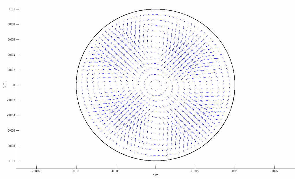
E_{213} magnetinis laukas, z=1/1 , t=T/4
