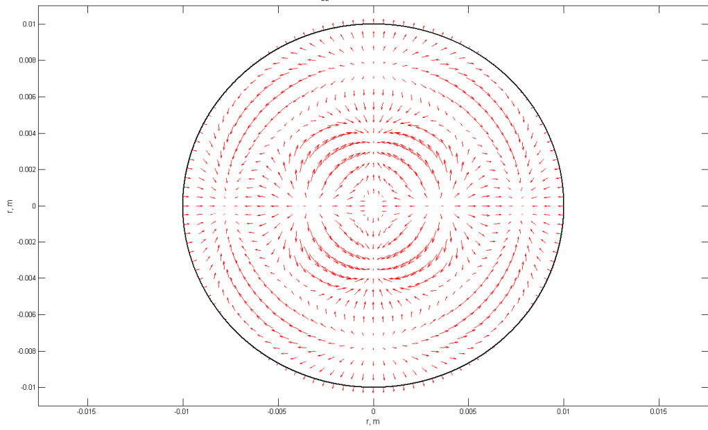
E_{z2} , elektrinis laukas, z=\lambda/4
