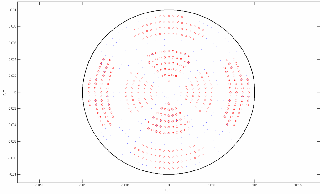
E_{z2} , elektrinis ir magnetinis laukai, z=\lambda/2
