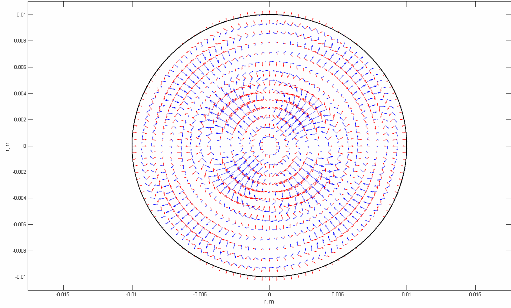
E_{z2} , elektrinis ir magnetinis laukai, z=\lambda/4
