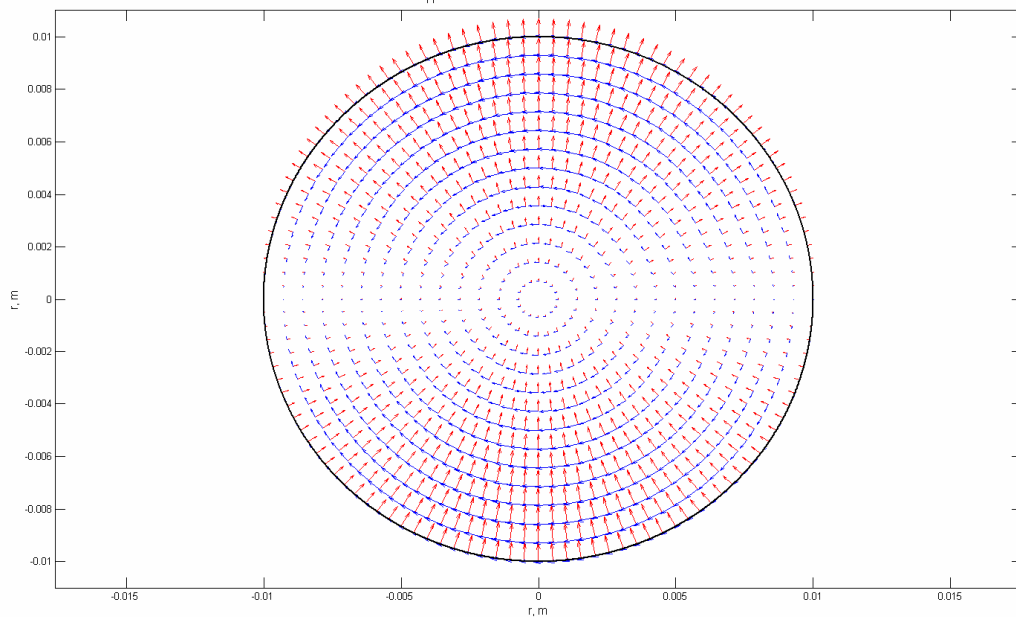
H_{11} , elektrinis ir magnetinis laukai, z=\lambda/4
