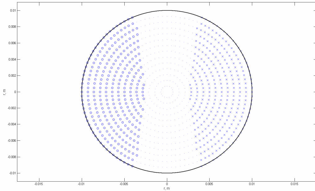
H_{11} , elektrinis ir magnetinis laukai, z=\lambda/2
