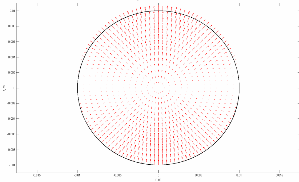
H_{11} , elektrinis laukas, z=\lambda/4
