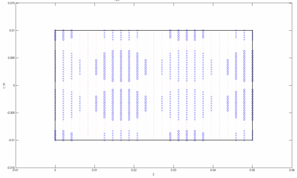
H_{123} elektrinis ir magnetinis laukai, \phi=90^\circ , t=T/4
