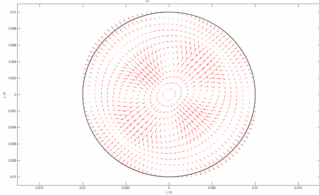
H_{22} , elektrinis laukas, z=\sqrt{4}
