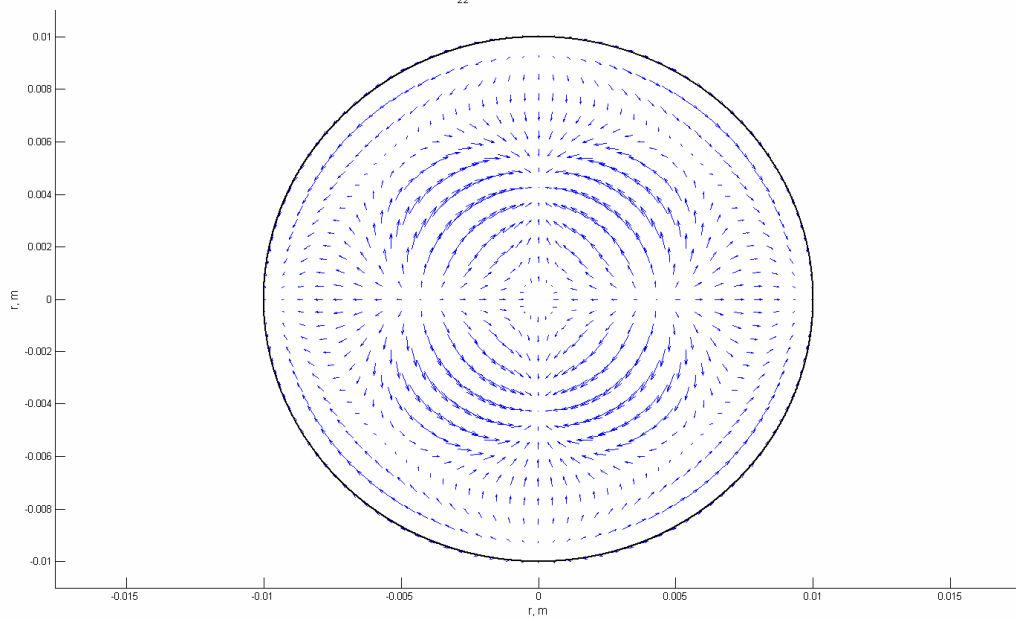
H_{z2} , magnetinis laukas, z=\lambda/4
