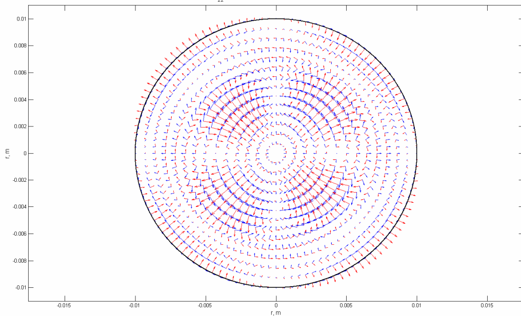
H_{z2} , elektrinis ir magnetinis laukai, z=\lambda/4
