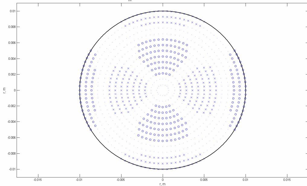
H_{22} , elektrinis ir magnetinis laukai, z=\sqrt{2}
